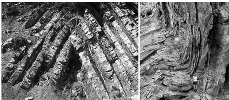
Изогнутые пласты
