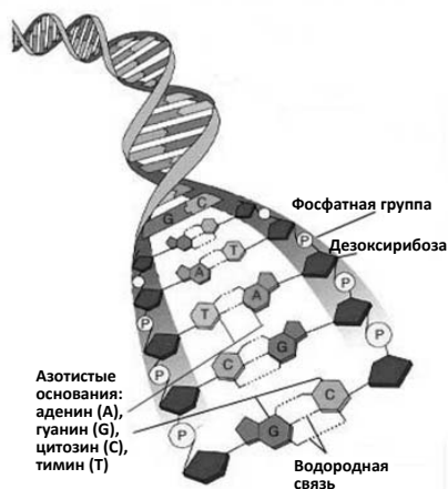
Структура ДНК.
